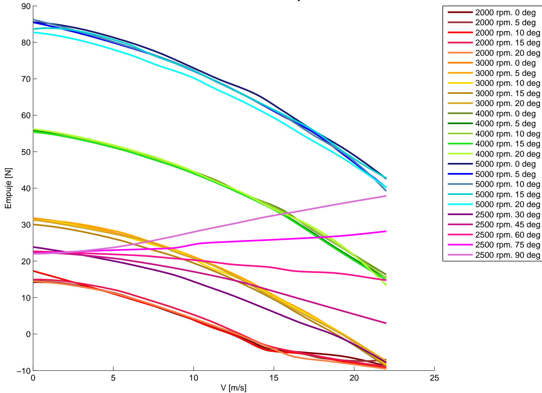
Tracción de la helice en cada ensayo
