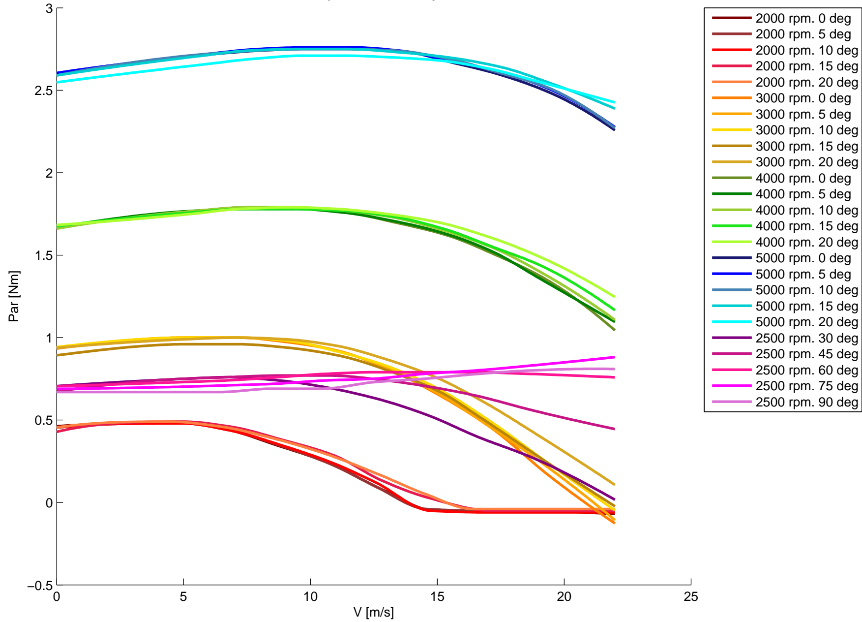
Torque en cada ensayo
